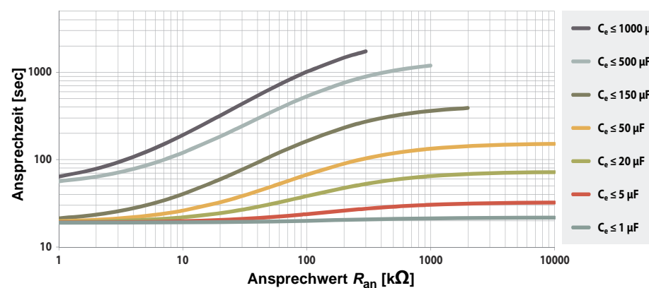
Ansprechzeit in Abhängigkeit von Ansprechwert und Netzableitkapazität nach IEC 61557-8 ( U_n = 690\text{ V} , f = 50\text{ Hz} ) Messbereich < 10\text{ M}\Omega
