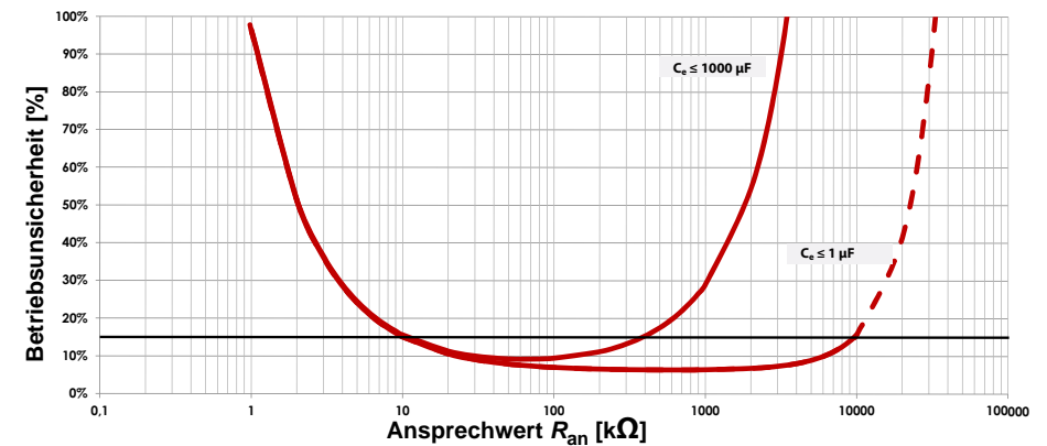
Prozentuale Betriebsmessunsicherheit in Abhängigkeit von Ansprechwert und Netzableitkapazität nach IEC 61557-8 ( U_n = 690\text{ V} , f = 50\text{ Hz} ) Messbereich < 10\text{ M}\Omega
