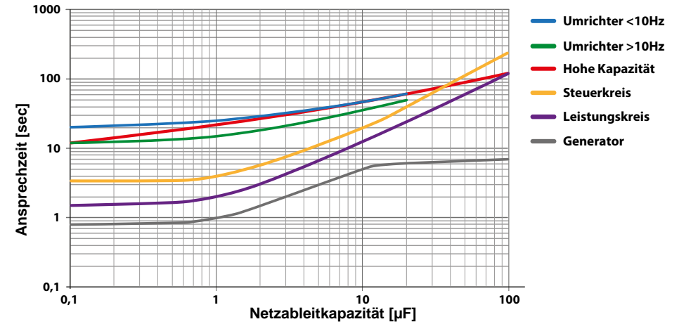
Typische Ansprechzeiten DC-Alarm bei RF in Abhängigkeit vom Messprofil und Netzableitkapazität
