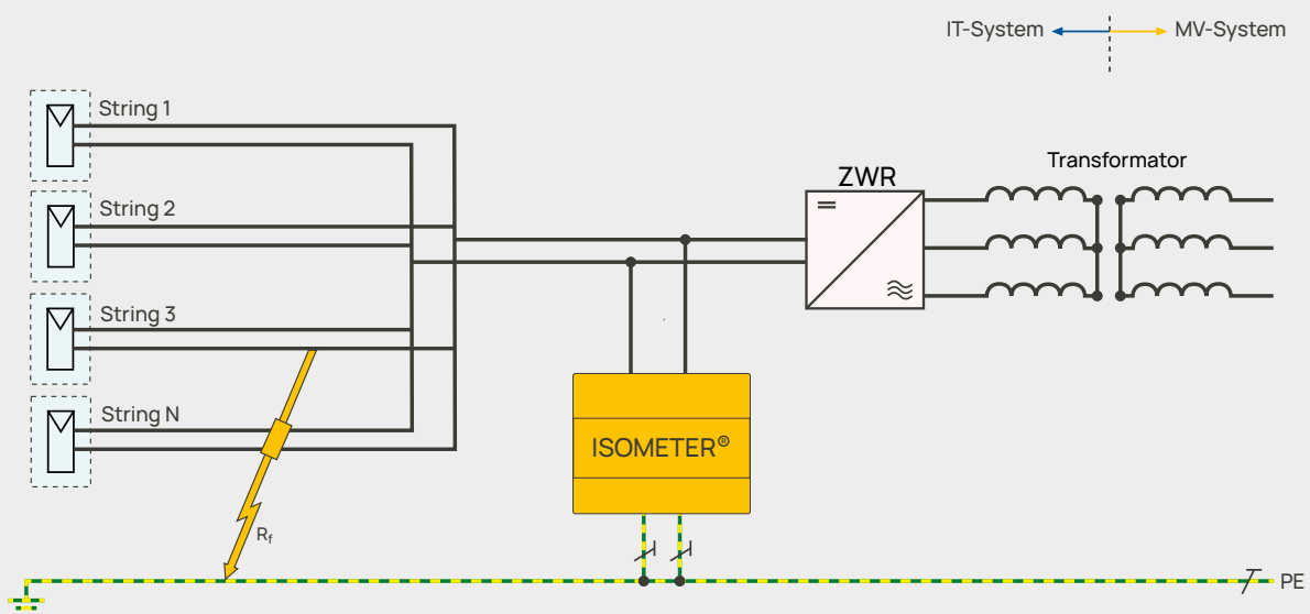
Bild 8: Zentralwechselrichter (ZWR)
